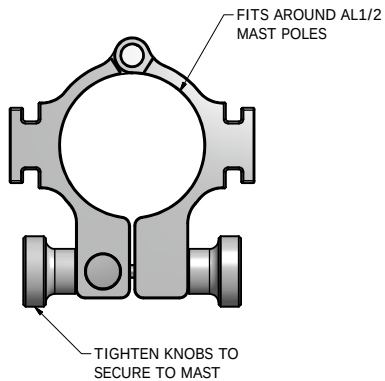
BSM2-P-A352-T00-000 POLE MOUNT-AL1/AL2-TWO WAY
