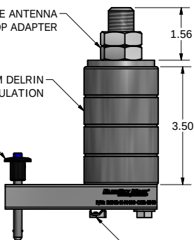
BSM2-K-M400-OE2-EM0 SIDE MOUNT-100 ARM-OE254 & COM201 ANTENNAS
