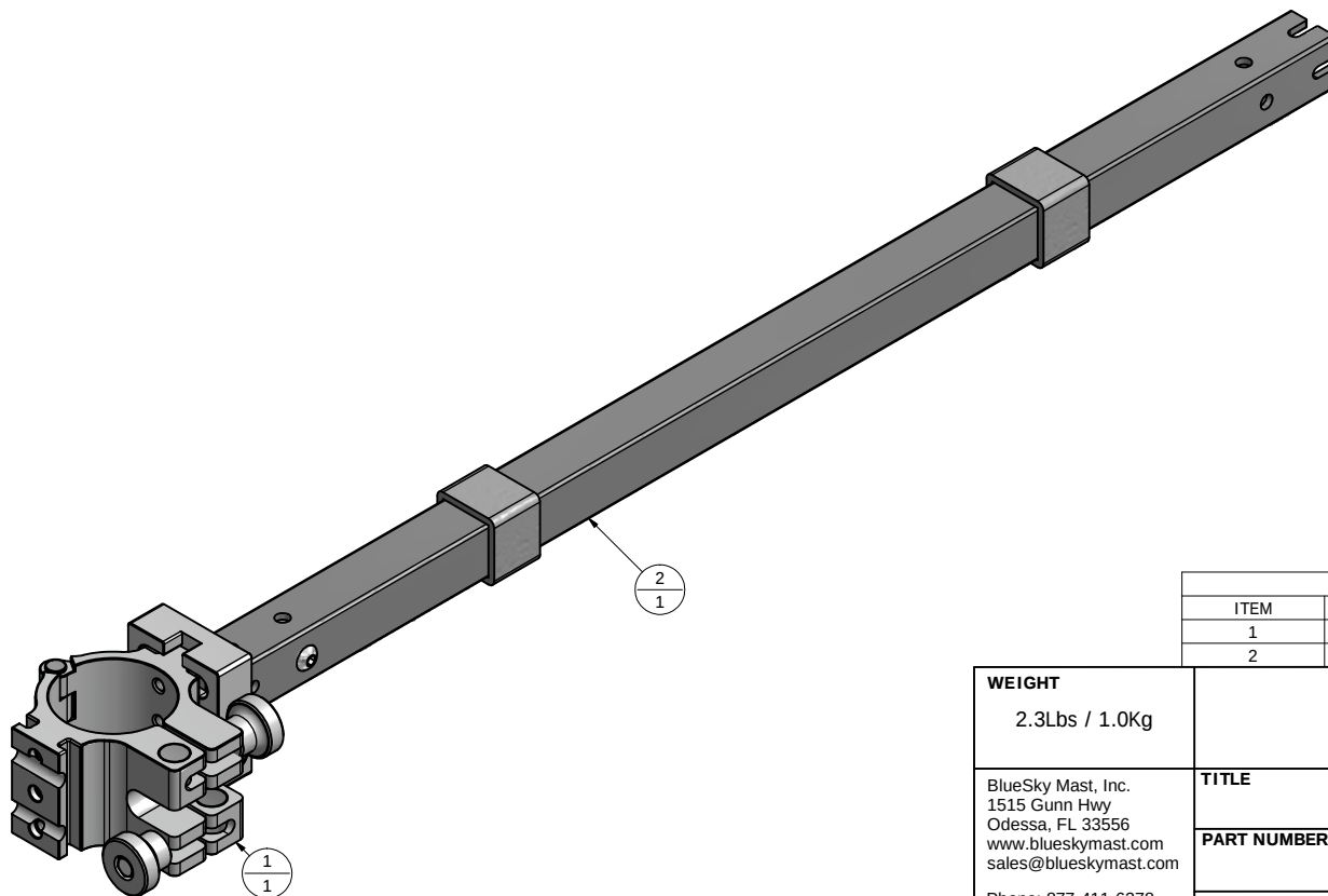
BSM2-P-A352-T00-000 POLE MOUNT-AL1/AL2-TWO WAY
