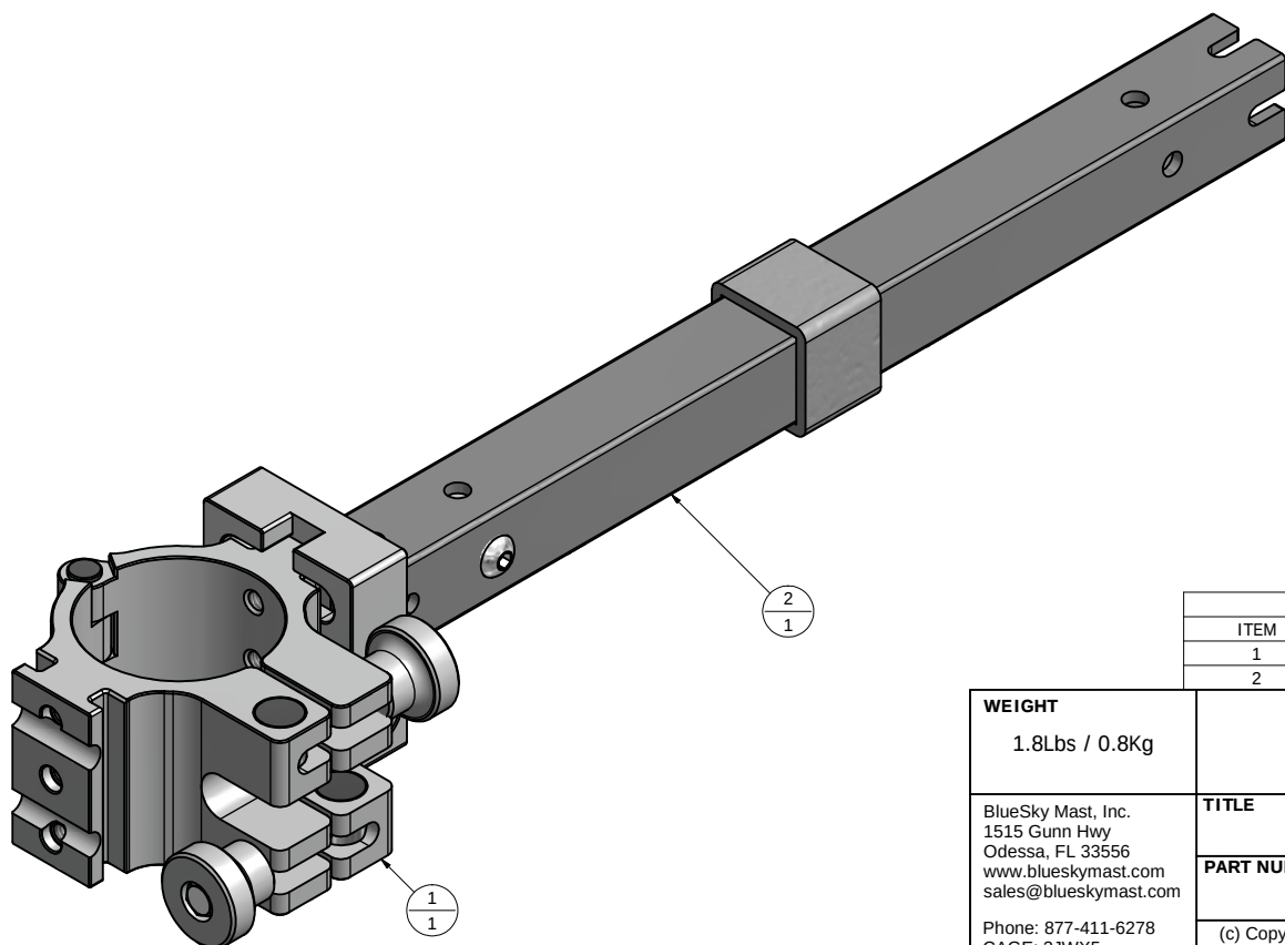
BSM2-P-A352-T00-000 POLE MOUNT-AL1/AL2-TWO WAY
