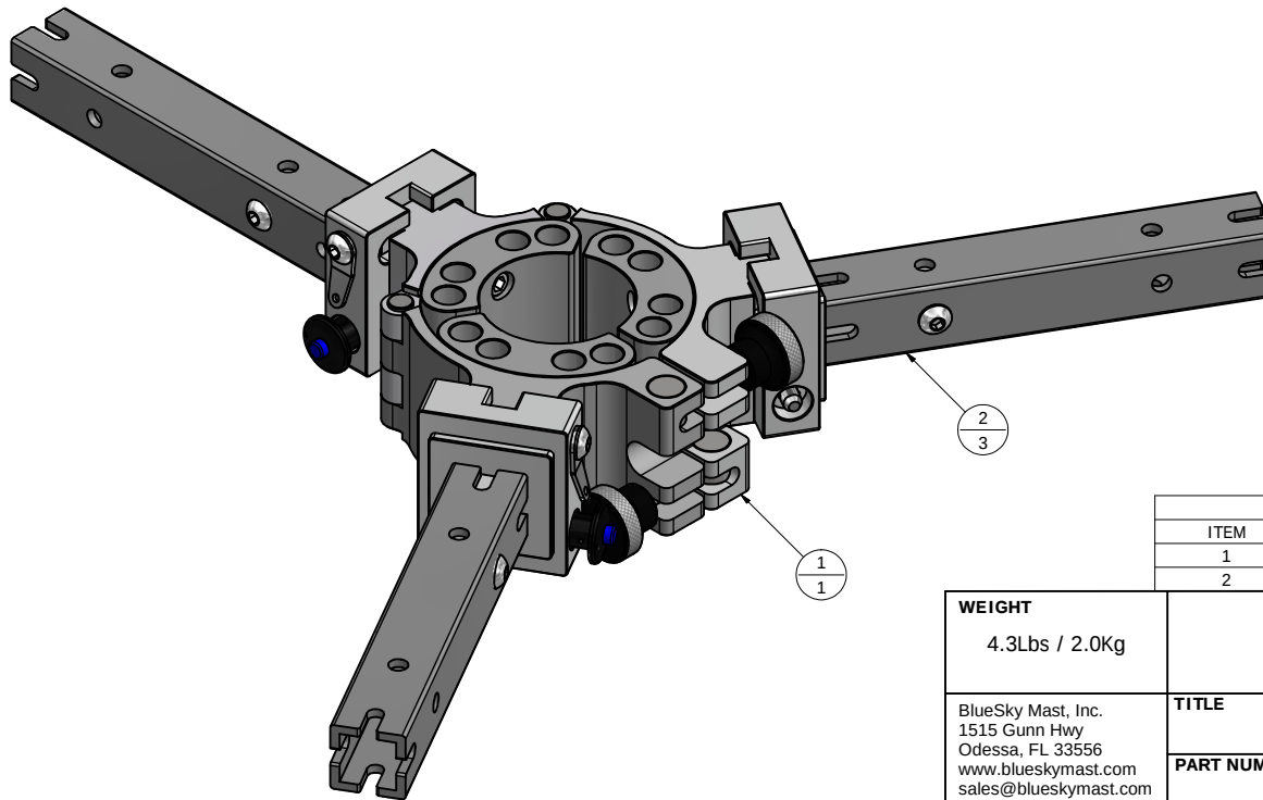
BSM2-P-A353-T00-000 POLE MOUNT-AL1/AL2-THREE WAY
