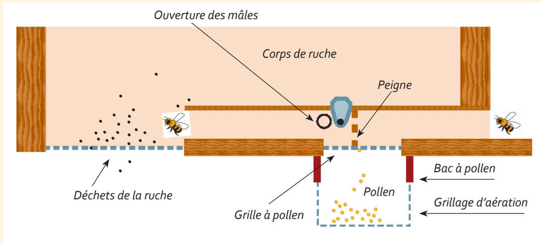
Les bacs de récolte sont maintenus par un clou situé à l'avant
