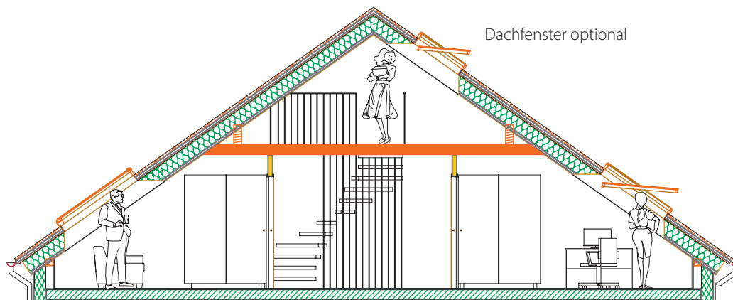
Dachausbau mit abgesenktem Spitzboden
