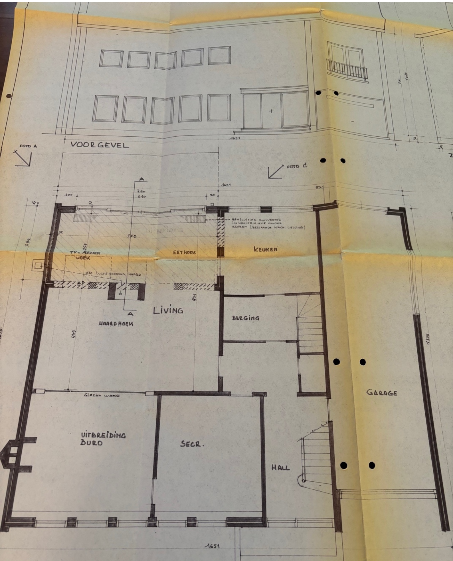
ALGEMEEN GRONDPLAN
