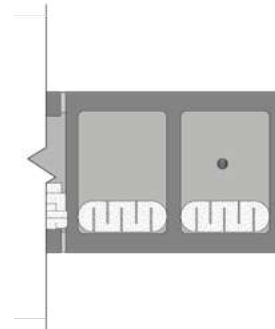
CMU 12×8×16 Jamb Unit
