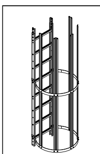
Lejdersektion med rygbøjle
