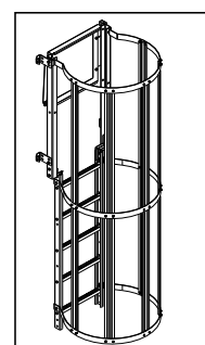
Topudstigning Lige frem incl. sikkerhedslåge
