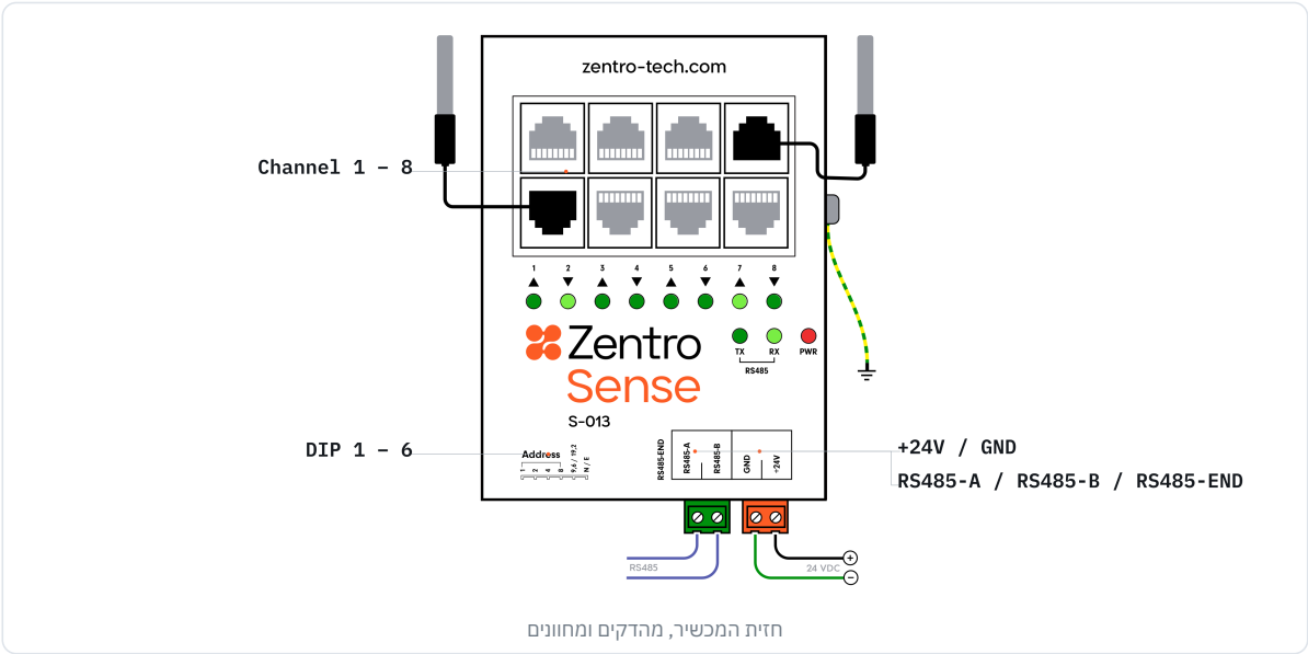
Channel1 1 – 8 מחברי RJ45 לחיישני טמפרטורה, חיישן אחד לערוץ
