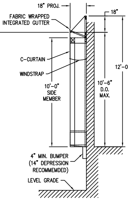
RIGHT SIDE ELEV.
