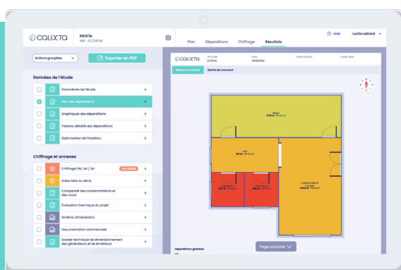
Plan du logement avec déperditions thermiques
