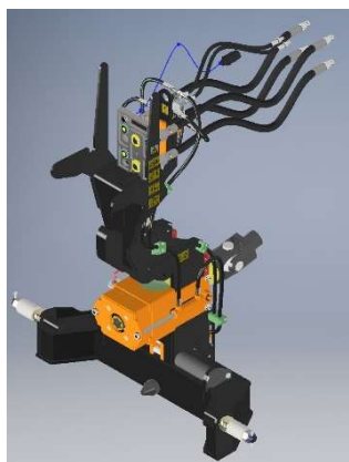
TM800-C3P Module tracteur avec PDF
