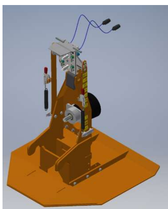
VMP800-K80 Module tracteur avec PDF
