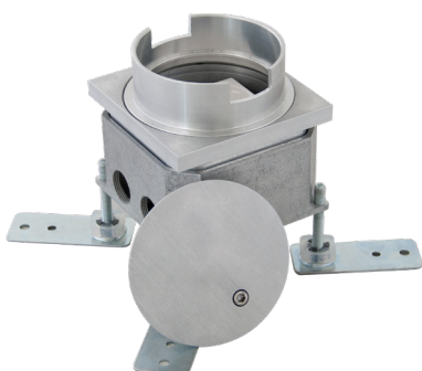
MASSO 8010 (CEE 16/5) - 840933
