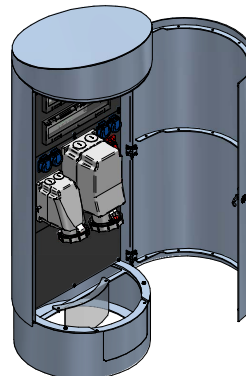
skap - 268441
