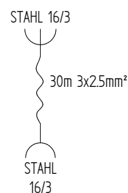
Type 573 «Stahl» – 860638
