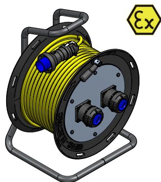
Type 573 «CEAG» – 860633
