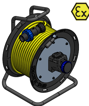
Type 573 «Stahl» – 860675
