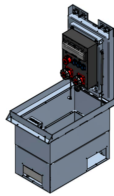
RONDO L - 260490
