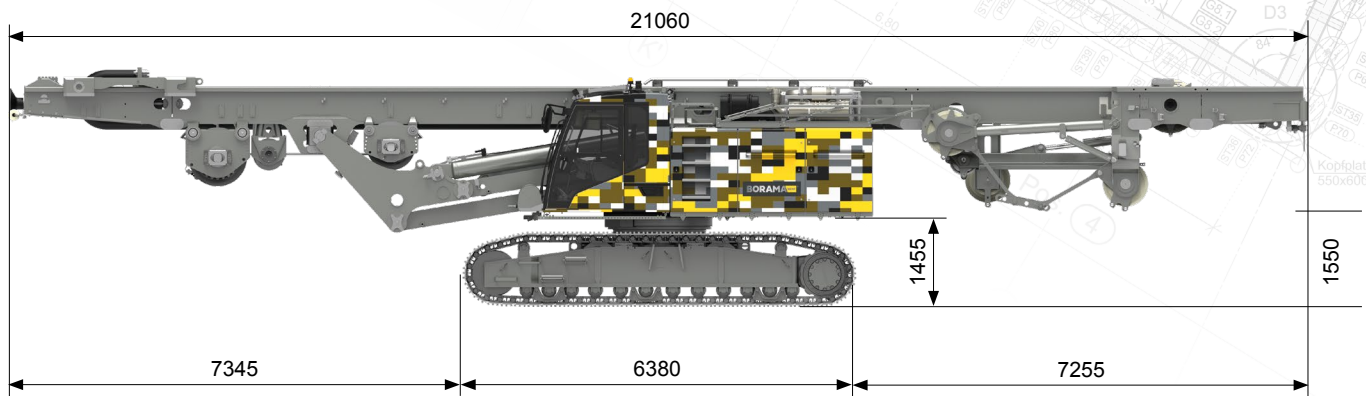
Transportstellung
