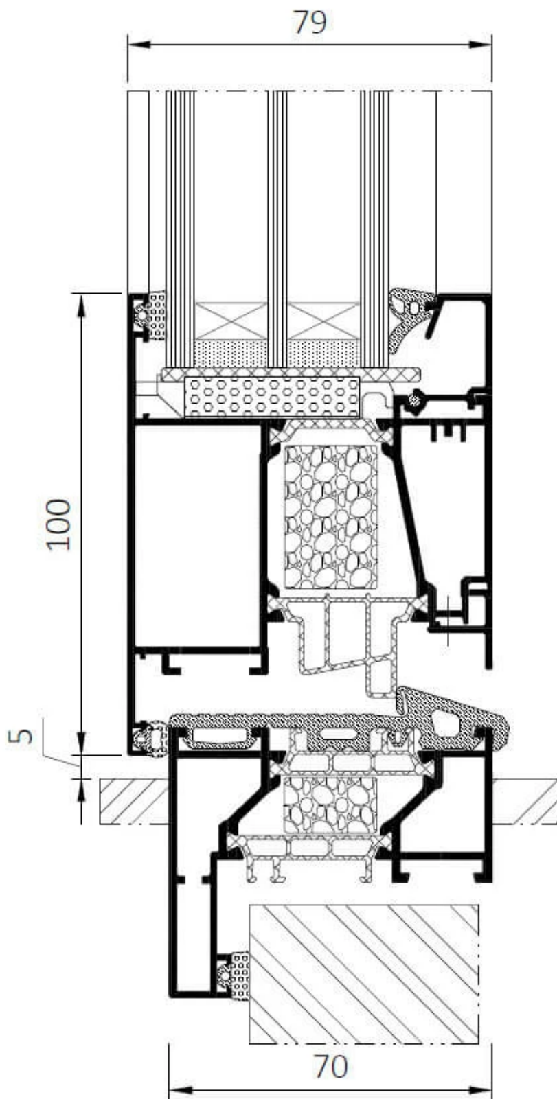
MB-79N Casement SI
