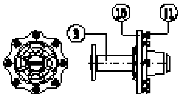
Løpenav for Gjødselvogn '94 Rammenr. etter 94-137
