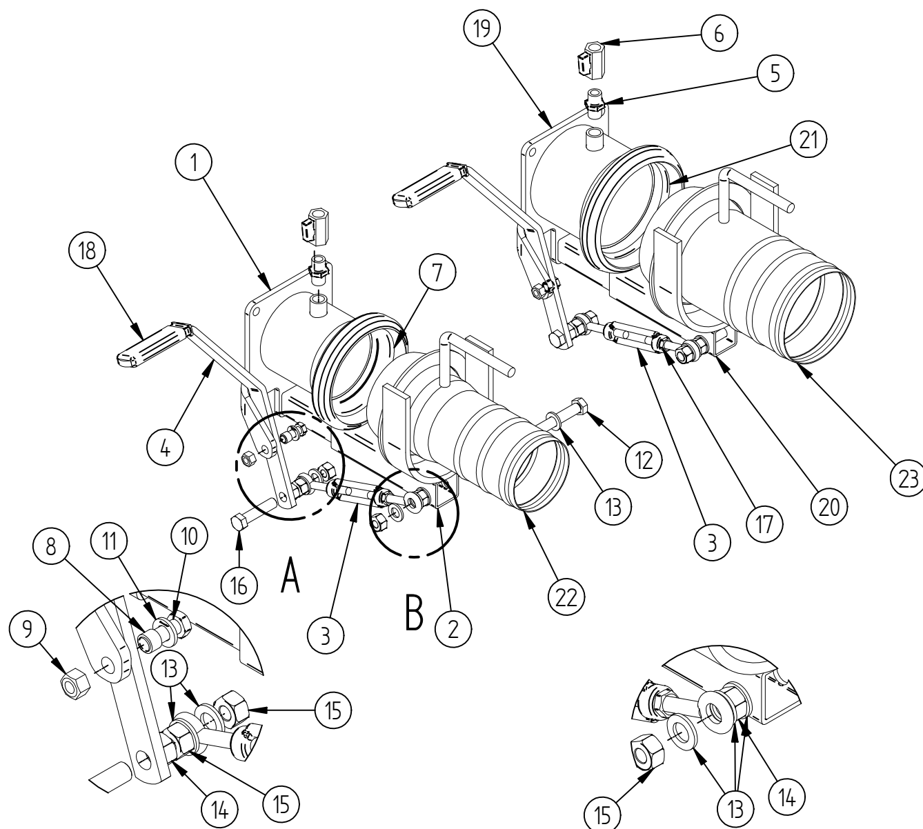
Detalj A
