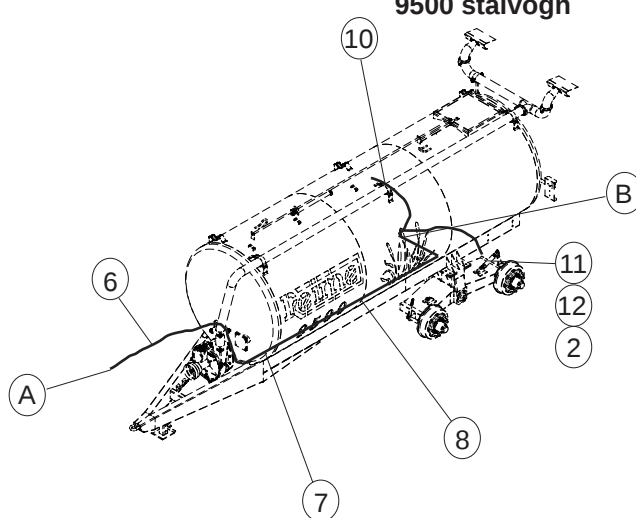
9500 stålvogn
