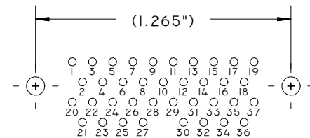
37 SOCKET
