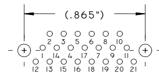
21 SOCKET
