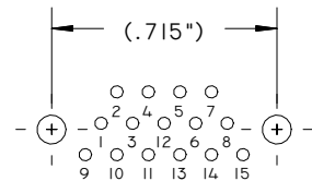
15 SOCKET
