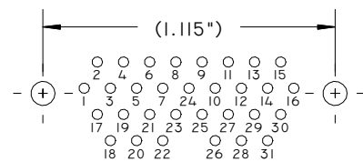
31 SOCKET
