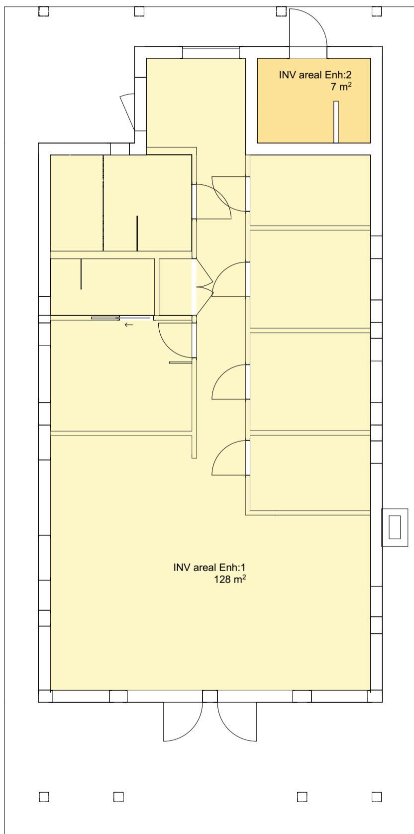
1:100 1. etasje
