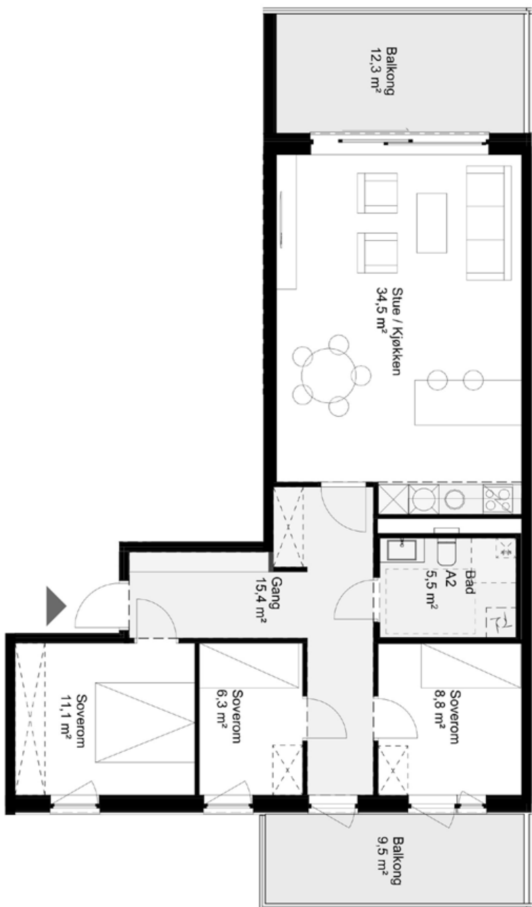
N13 Plantegning
