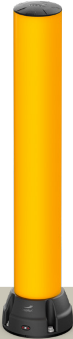
BO170B >>> 7,5 kJ
