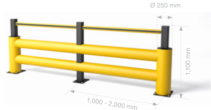
TB 400 DOUBLE PLUS 39.10 kJ
