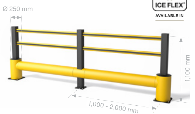
TB 400 PLUS 20.10 kJ
