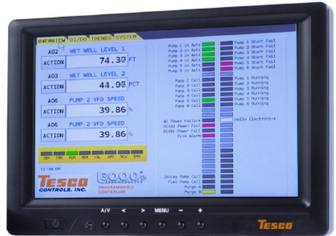
Door mount HDMI
