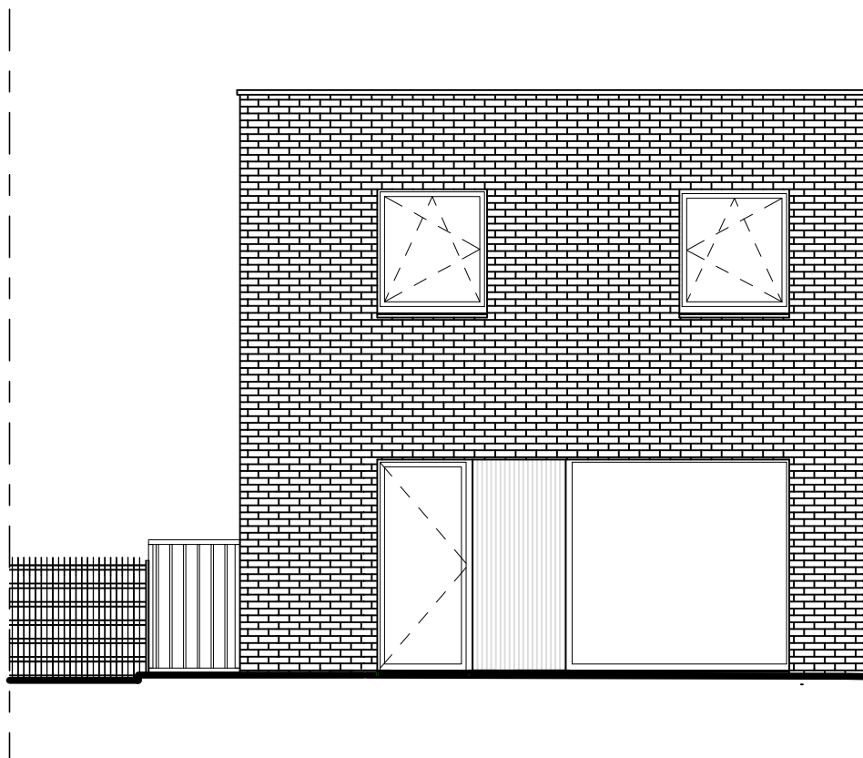
Vorgevel
