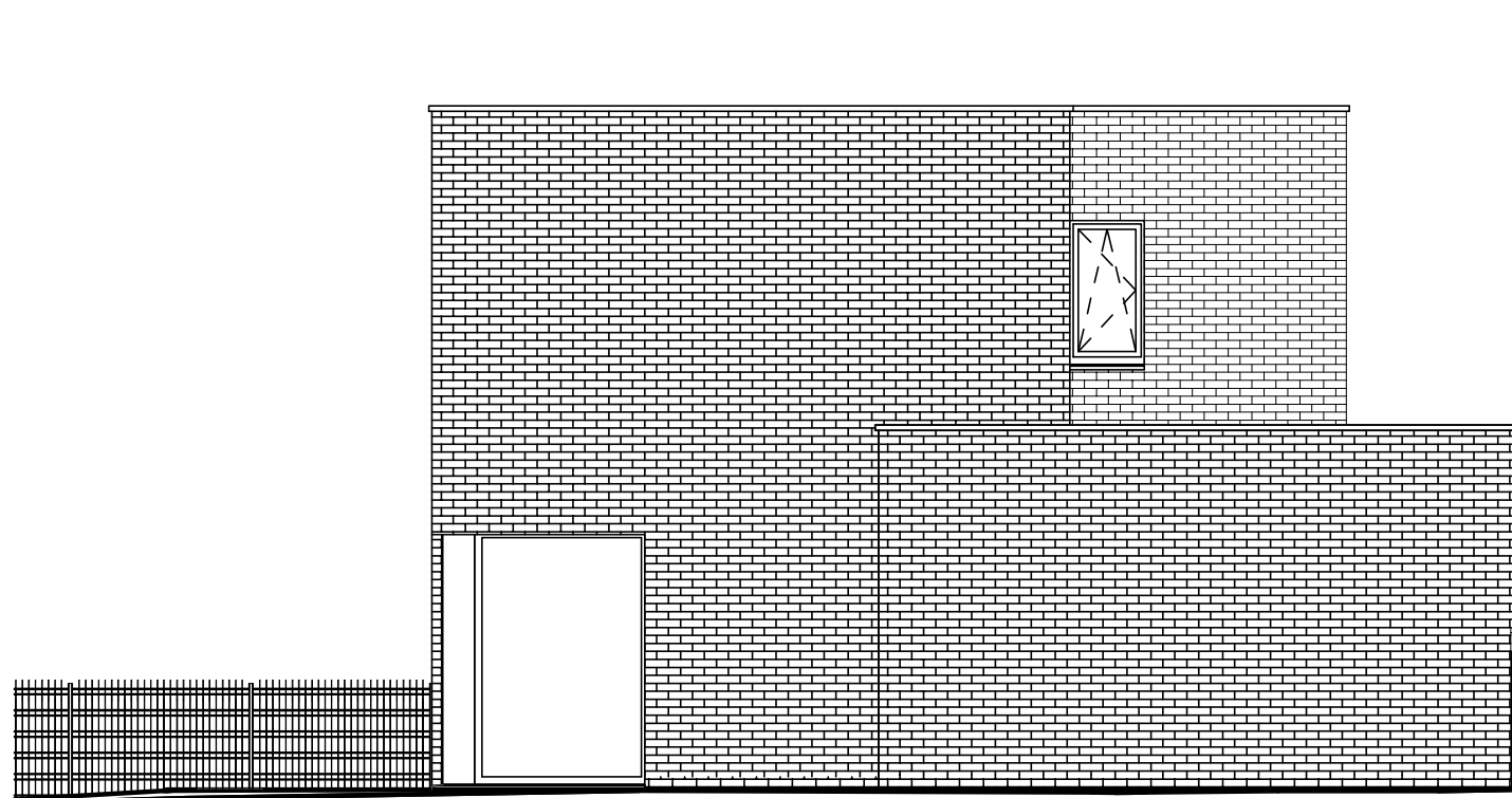
Linker zijgevel
