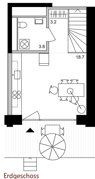
GRUNDRISS WOHNUNGSTYP
