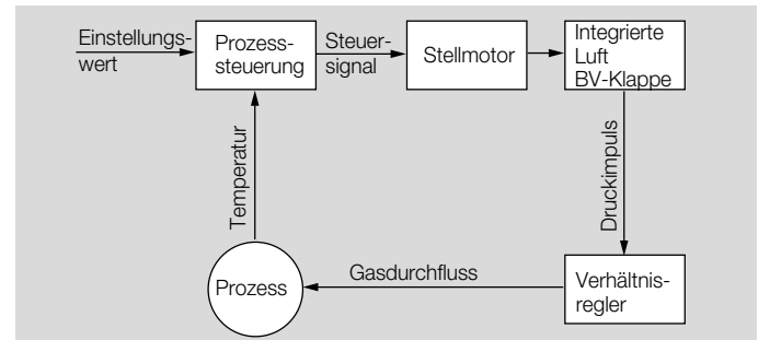
Basisregelkreis
