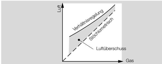
Luft-/Gasmenge
