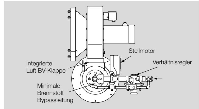
Grundlegende Brennerkomponenten
