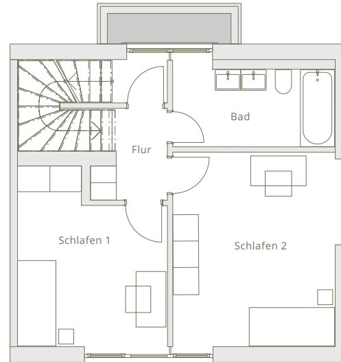
OBERGESCHOSS
