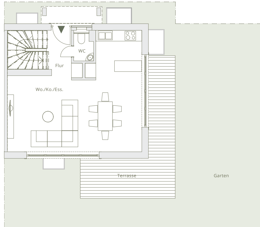
ERDGESCHOSS
