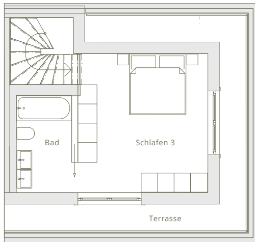
DACHGESCHOSS
