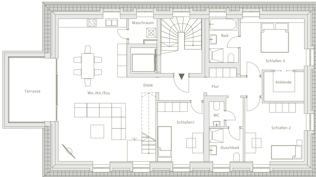
DACHGESCHOSS
