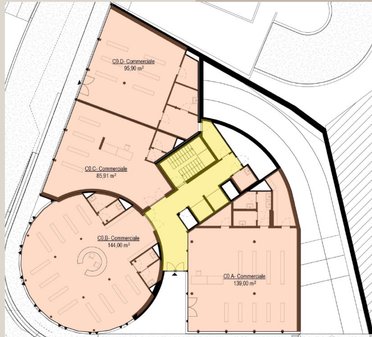
ERDGESCHOSS - ANORDNUNG DER GESCHÄFTSRÄUME
