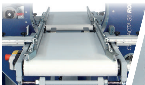
CONVOGLIATORE ORIZZONTALE A NASTRI MOTORIZZATI REGOLABILE IN LARGHEZZA HORIZONTAL MOTORIZED BELT CONVEYORS ADJUSTABLE IN WIDTH
