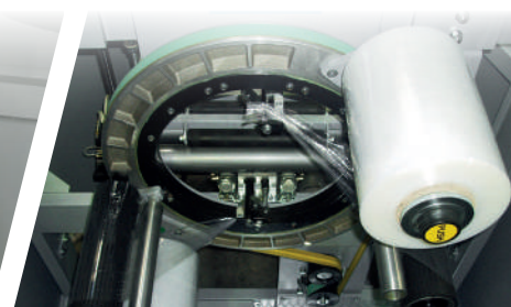
GRUPPO PORTABOBINA FILM CARRIAGE
