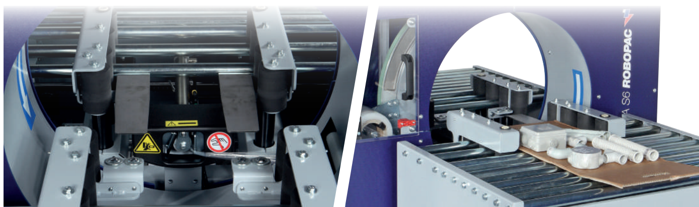
CONVOGLIATORE A RULLI VERTICALI MOTORIZZATI, REGOLABILI MANUALMENTE IN LARGHEZZA E DETTAGLIO GRUPPO PINZA E TAGLIO. VERTICAL MOTORIZED ROLLERS CONVEYORS, MANUAL WIDTH ADJUSTABLE/ CLAMPING-CUTTING DETAIL.
