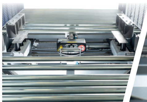
CONVOGLIATORE A RULLI FOLLI E GUIDE MOTORIZZATE VERTICALI (regolabili in larghezza) IDLE ROLLER CONVEYORS AND VERTICAL MOTORIZED GUIDES (adjustable width)
