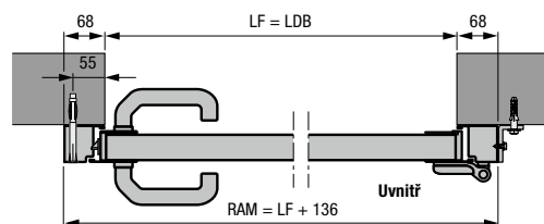
Vedlejší dveře s hliníkovou blokovou zárubní, profil typu 2 Montáž za otvorem
