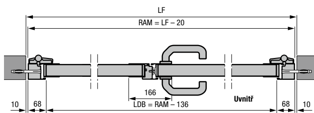
Dvoukřídle vedlejší dveře s hliníkovou blokovou zárubní, profil typu 2 Montáž v otvoru
