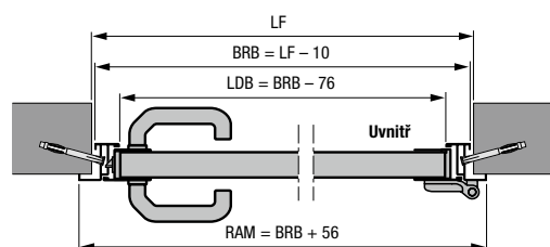
Vedlejší dveře s hliníkovou rohovou zárubní, profil typu 2 Vnitřní doraz
