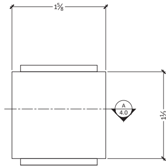
1 Post Cap - Top View SCALE: 1:1
