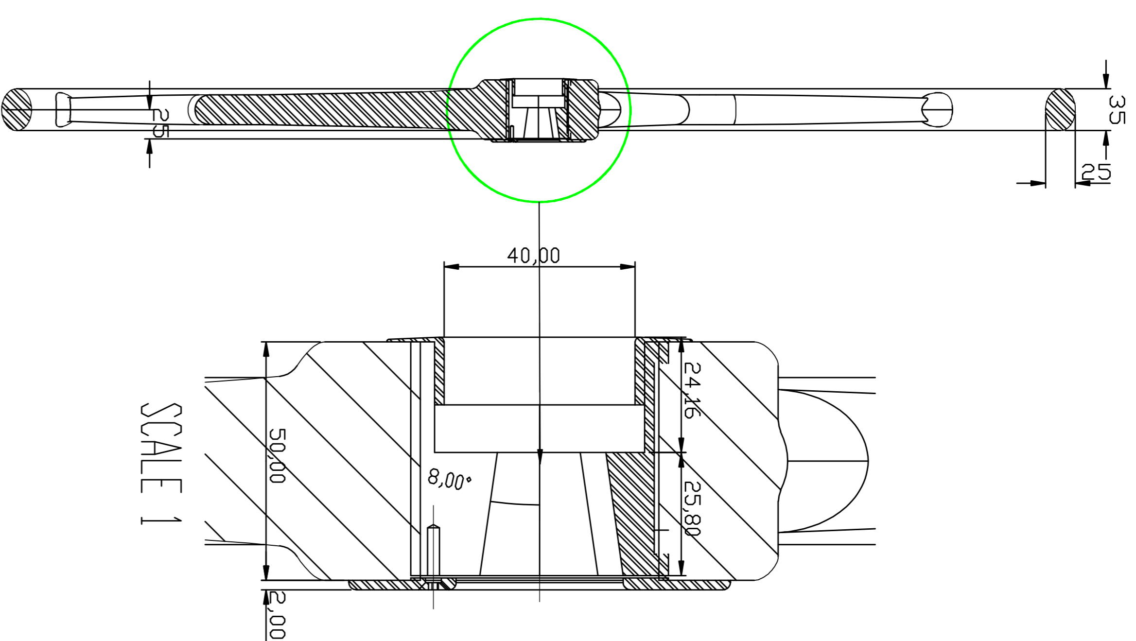
SECTION A-A
