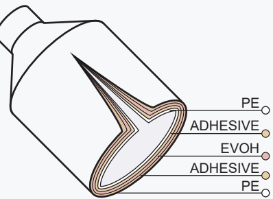
5 LAYER TUBE
