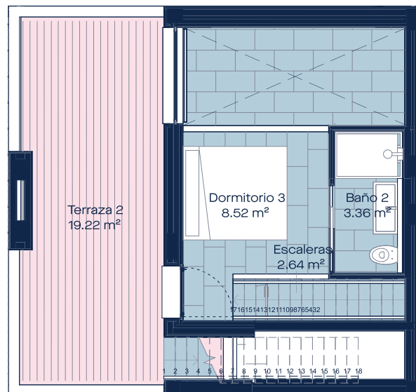
Planta Primera / FIRST FLOOR
