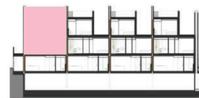
Sección Bloque 2
