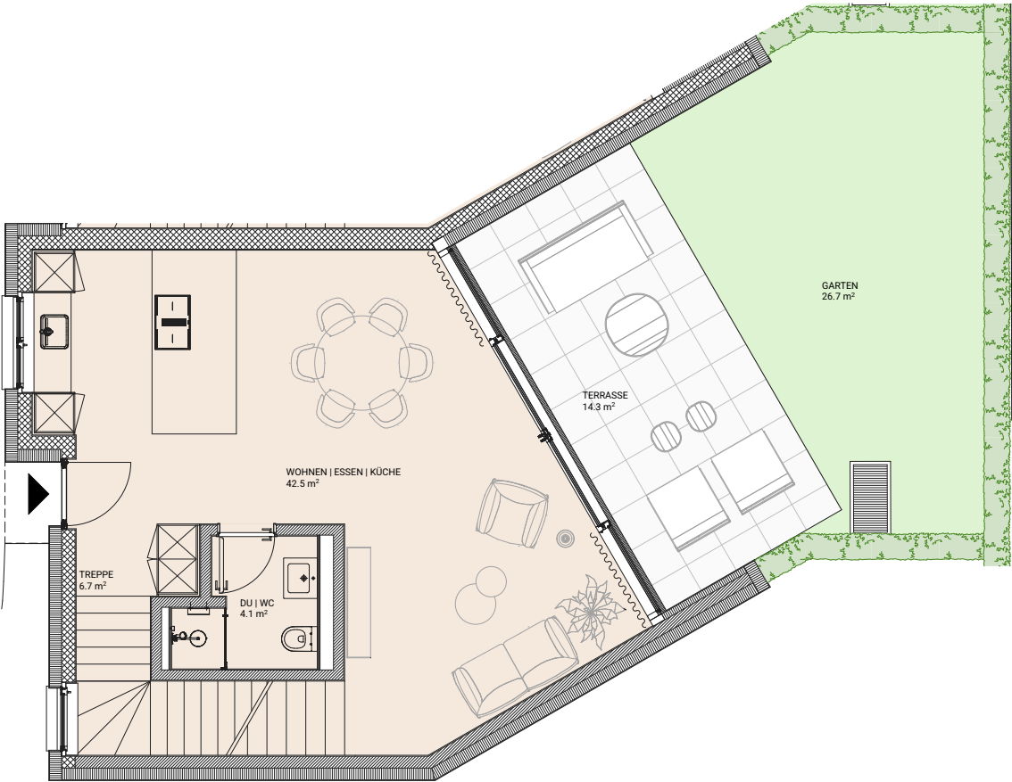
ERDGESCHOSS
