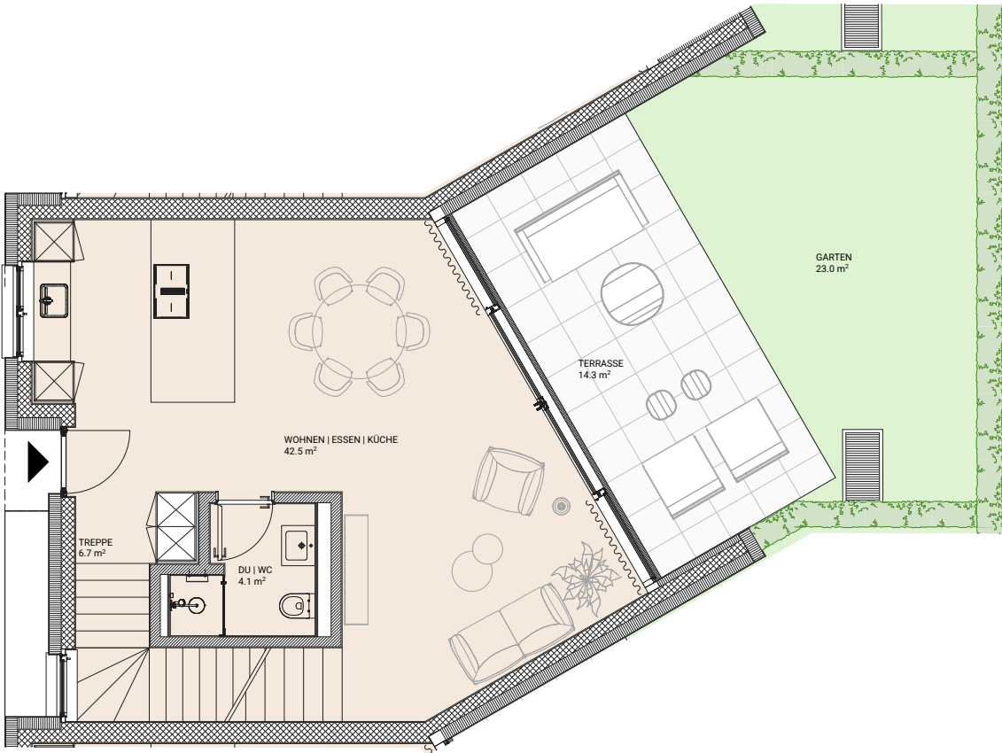
ERDGESCHOSS
