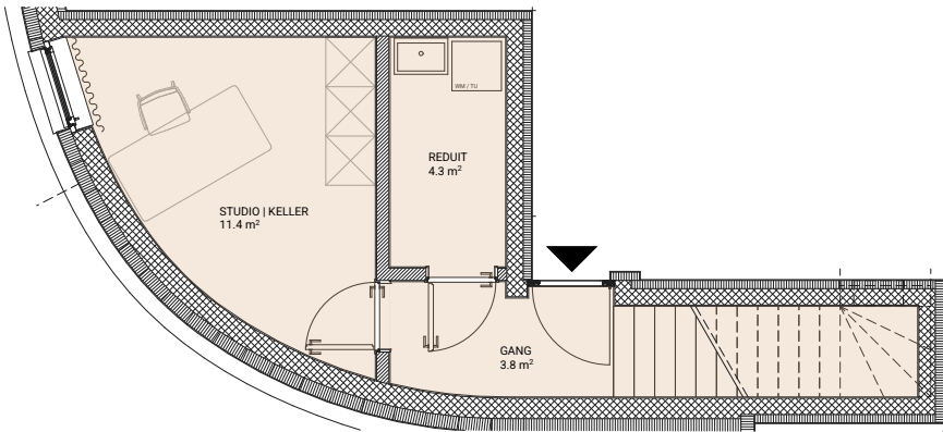
UNTERGESCHOSS
