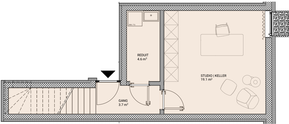
UNTERGESCHOSS
