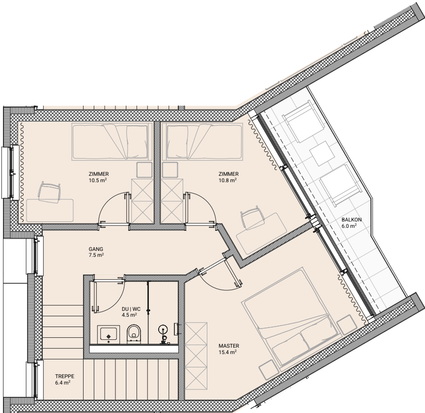
OBERGESCHOSS
