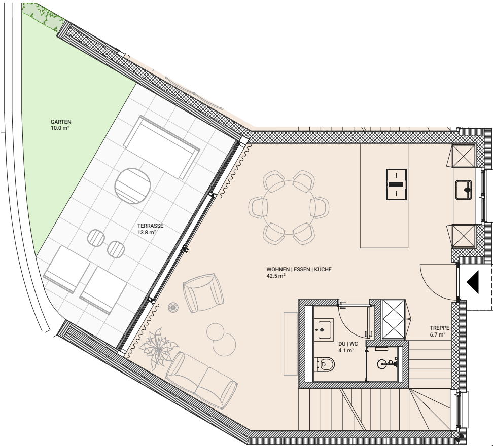
ERDGESCHOSS
