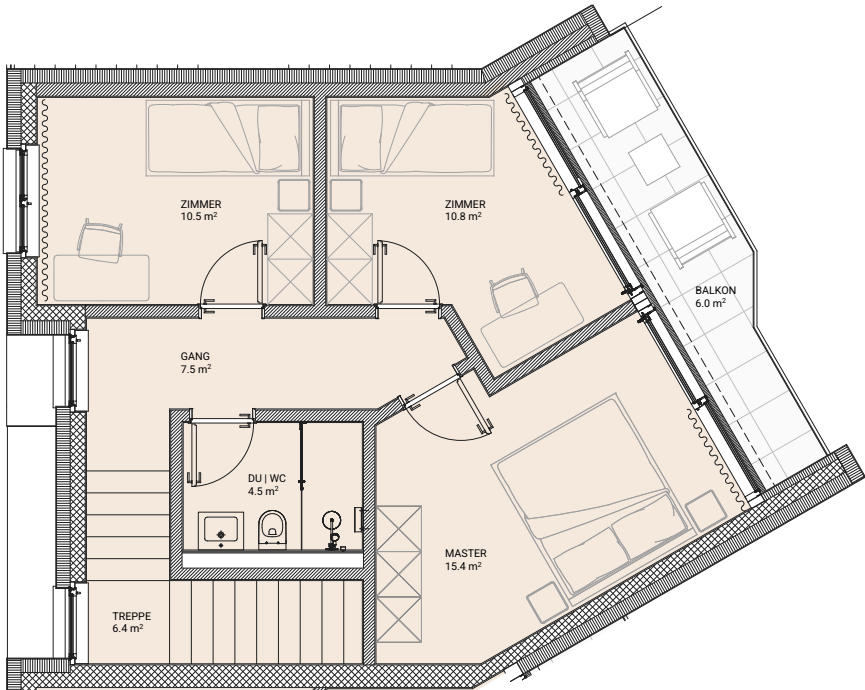
OBERGESCHOSS
