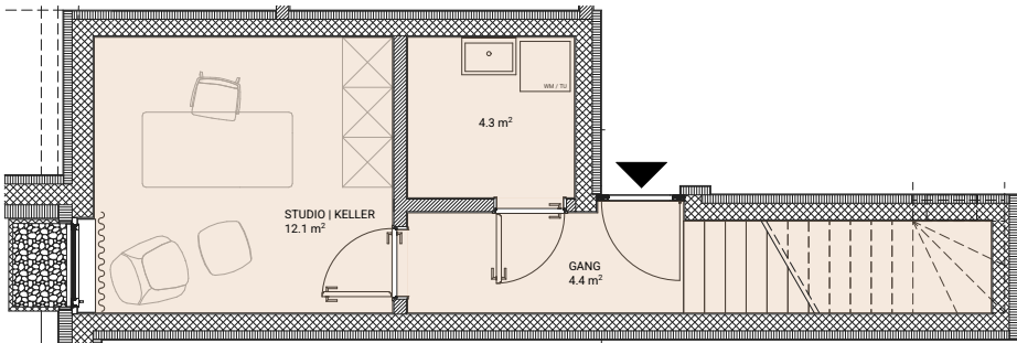
UNTERGESCHOSS
