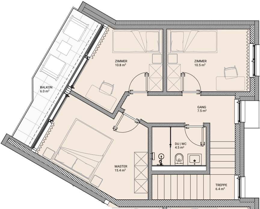
OBERGESCHOSS
