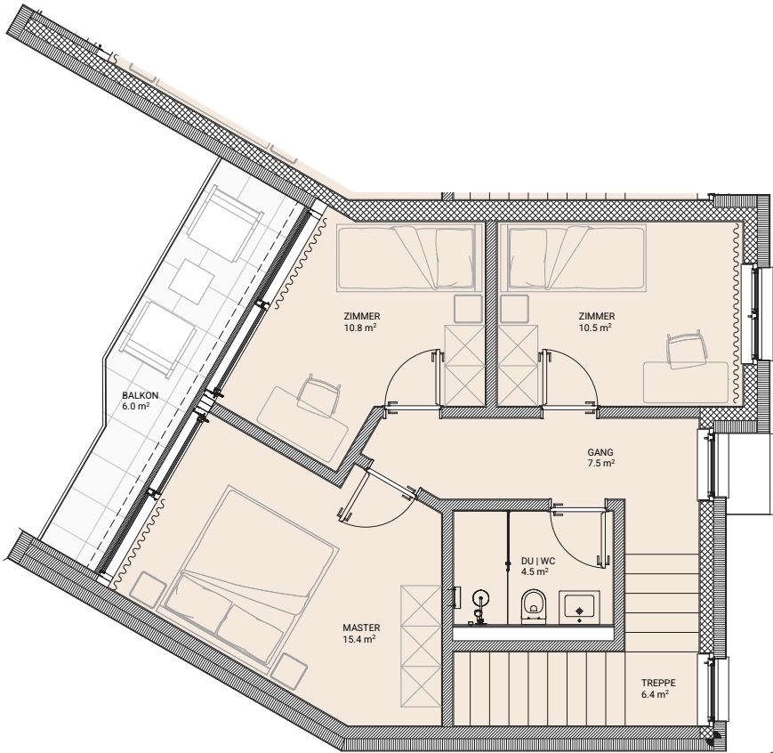
OBERGESCHOSS
