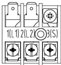
bornier d'alimentation de l'unité intérieure
