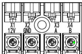
Bornier de signal
