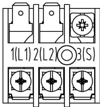
bornier de raccordement des unités intérieure et extérieure
