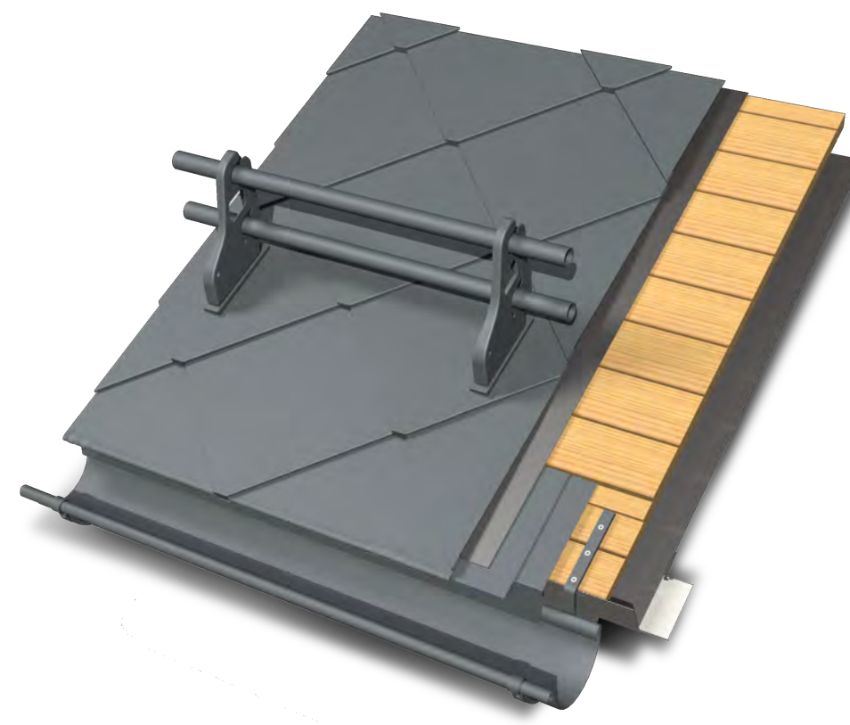
DETAIL SCHNEEFANG
