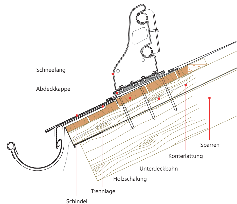
DETAIL SCHNEEFANG
