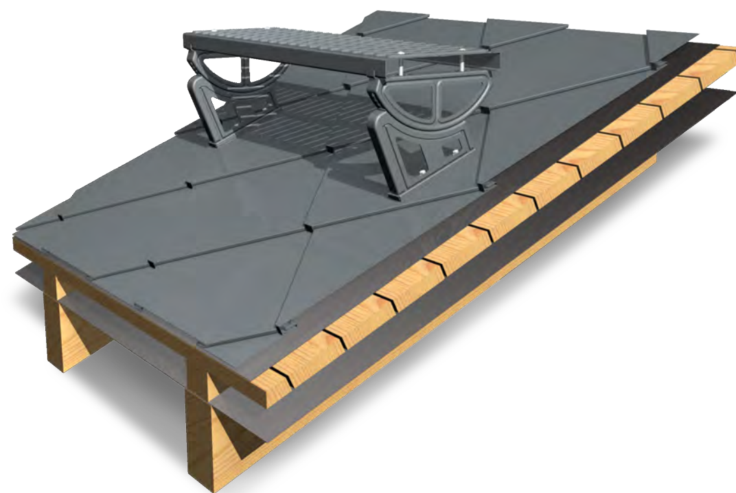
DETAIL LAUFROST
