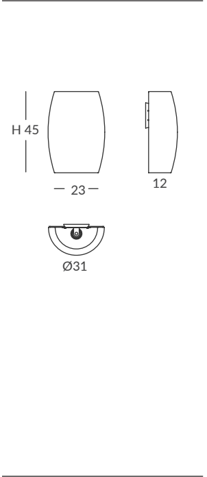
WALL LAMP / APLIQUE IP20
