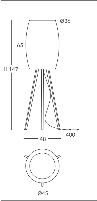
FLOOR LAMP / PIE DE SALÓN IP64
