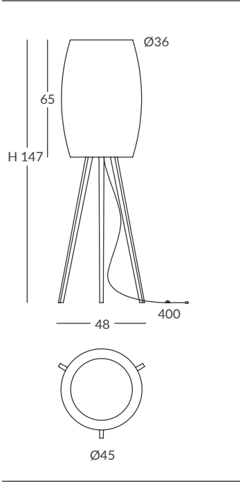
FLOOR LAMP / PIE DE SALÓN IP20
