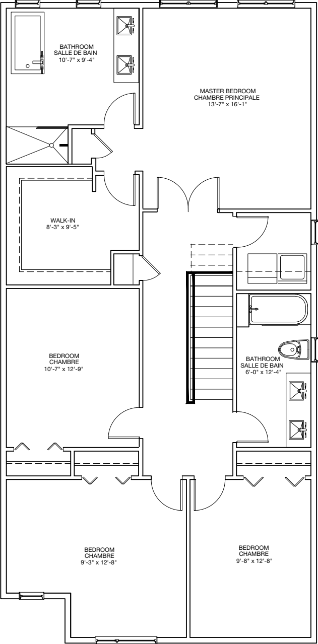
2 nd floor 2 e étage
