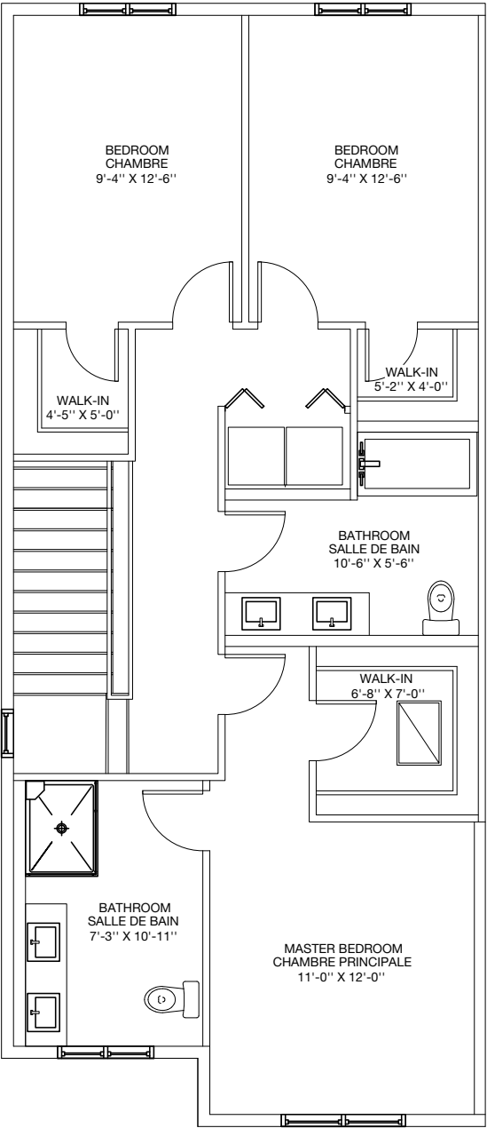
2 nd floor 2 e étage
