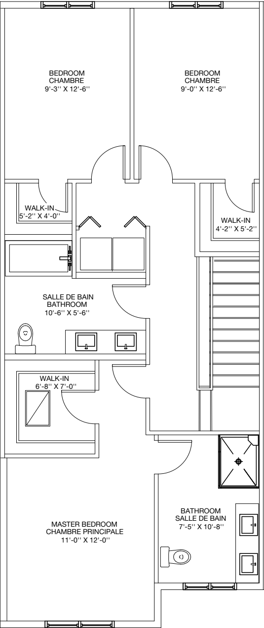
2 nd floor 2 e étage
