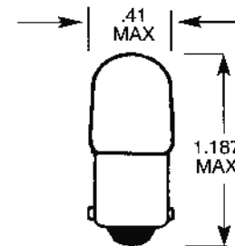
T-3.25 MINIATURE BAYONET
