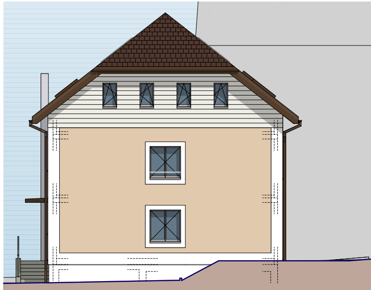
FACADE NORD
