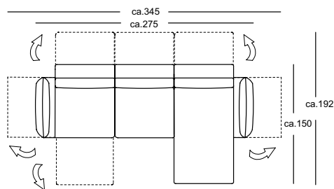
L-ASO-ES 386/175 le. ASS-PSZ 386/100 ri.
