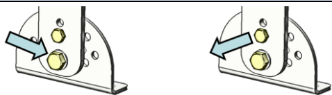
Boulon de pivotement Boulon de verrouillage
