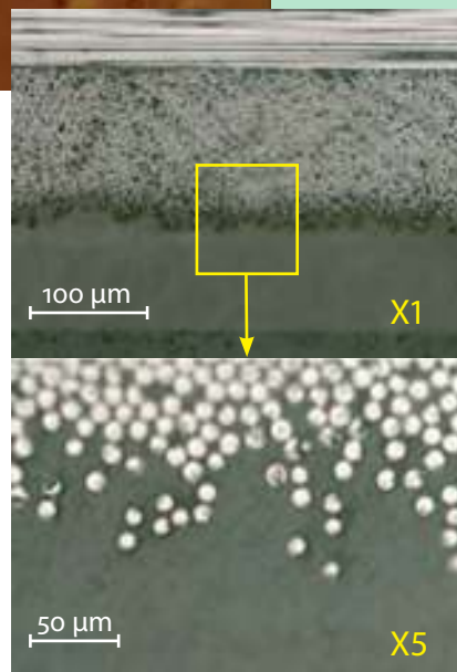
Phasengrenzsbereich zwischen Duroplast- und Thermoplastfolie
