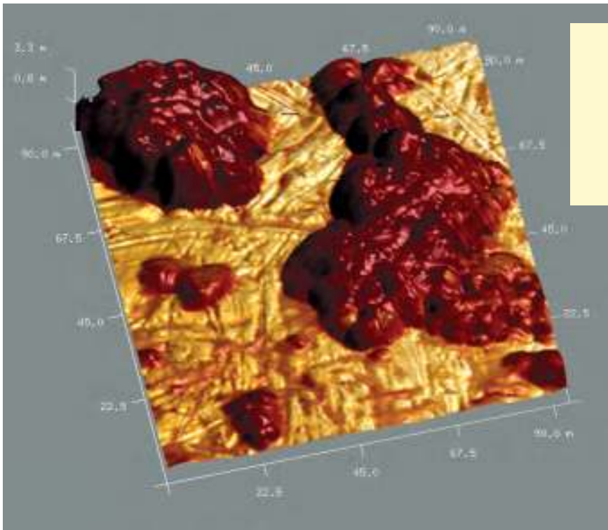
3D Topographie und E-Modul-Karte eines Transferfilms
