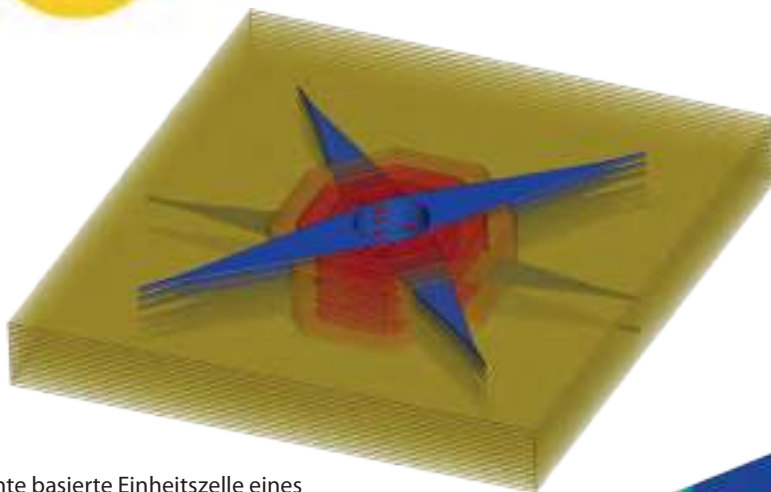
Finite-Elemente basierte Einheitszelle eines Mehrschichtverbundes mit Faserumlenkungsbereich
