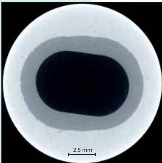
μCT-Aufnahme eines neuen Stators
