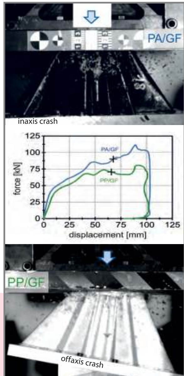
Inaxis und Offaxis Crashtest von Organoblech-Crashabsorber
