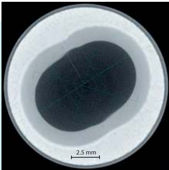
μCT-Aufnahme eines Stators nach Dosierung von Nanopartikelsuspensionen (TiO 2 )
