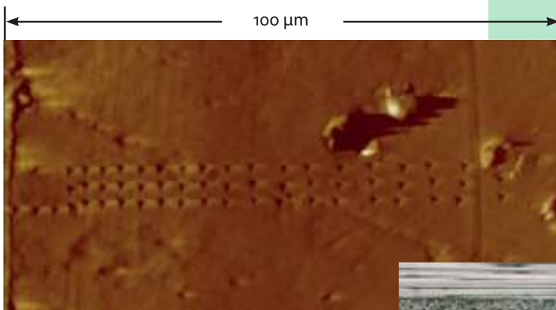
Aufnahme der Nano-Indentierung der Thermoplast- (links) und Duroplastzone (mit Faserreststücken, rechts)
