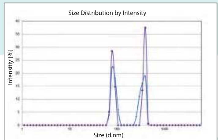
Partikelgröße-Verteilung von gefriergetrockneten und redispersierten Nanopartikeln
